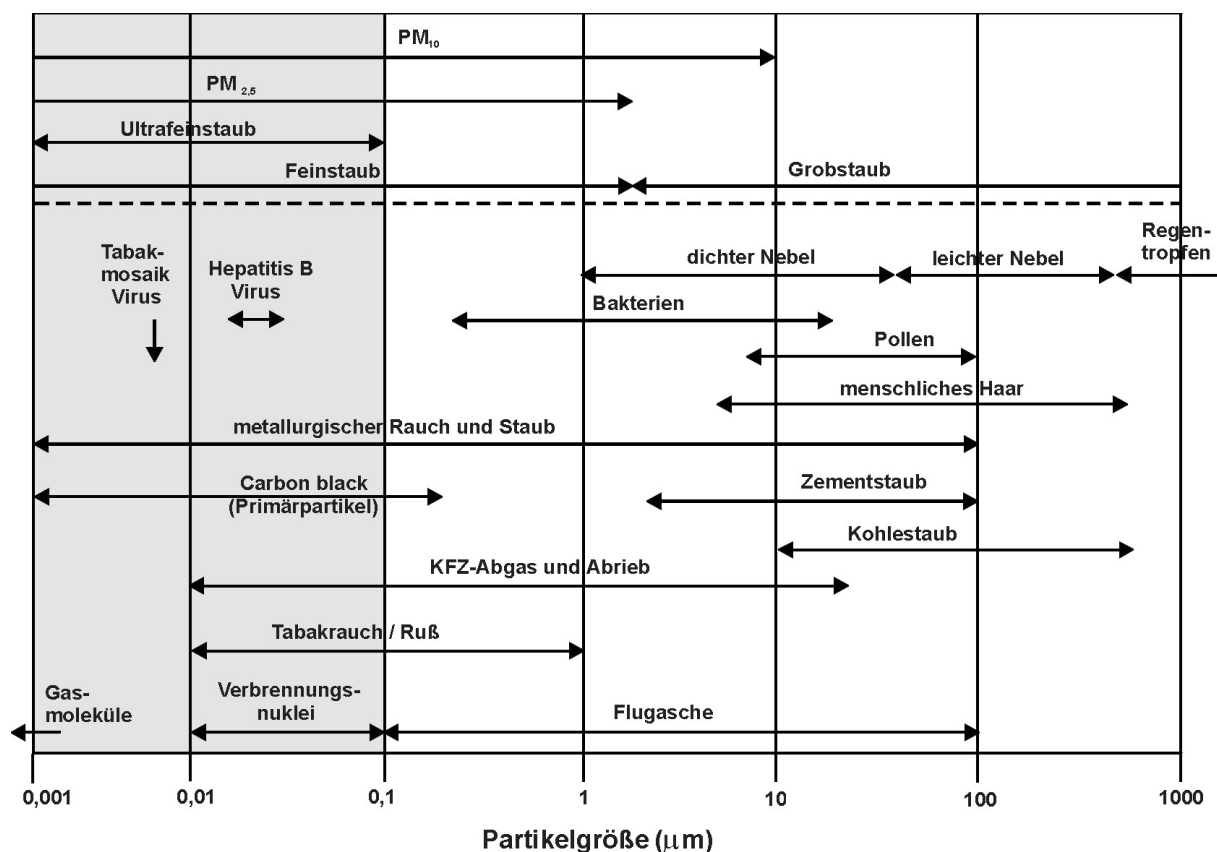
Abb.1: Partikeldefinitionen und Größenbereiche umweltrelevanter Partikel [Krug 2003]
